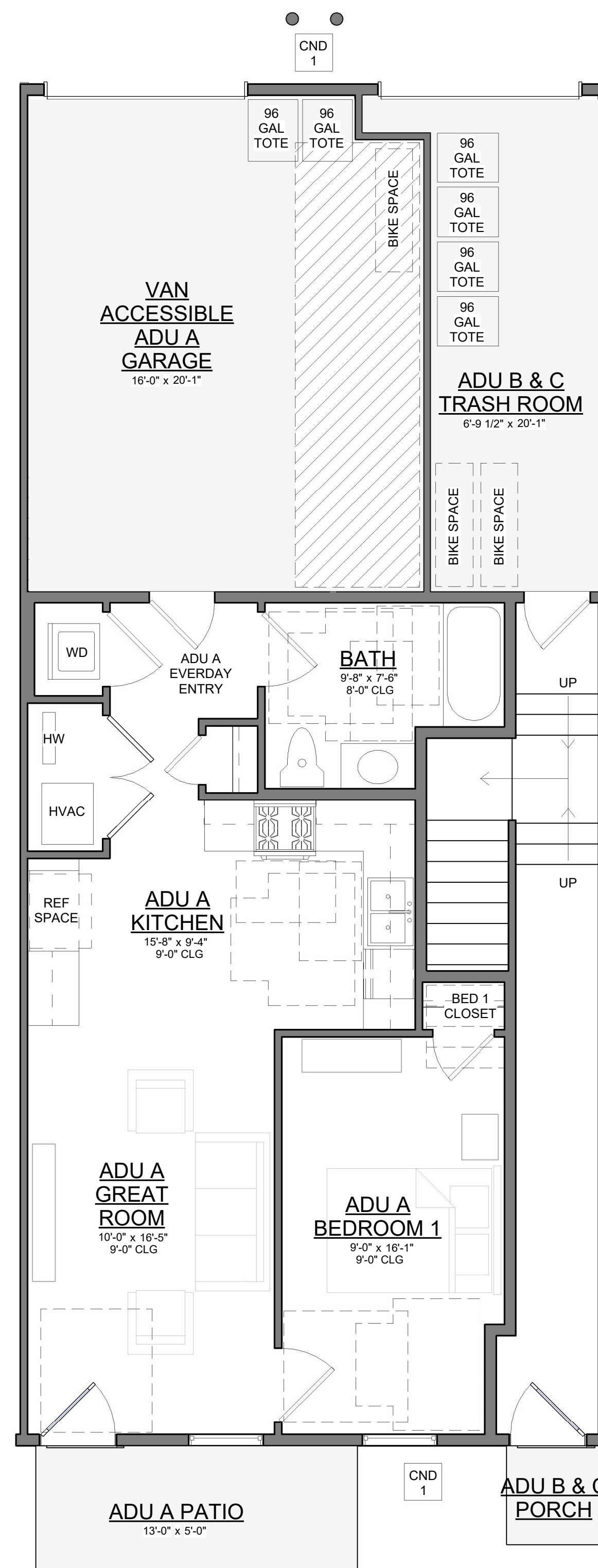
ADU A - VAN ACCESSIBLE GARAGE
